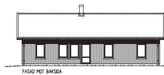
FASAD MOT BAKSIDA
