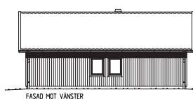
FASAD MOT VÄNSTER
