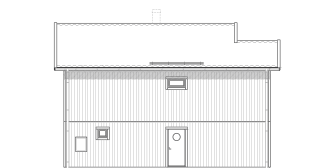
FASAD MOT BAKSIDA
