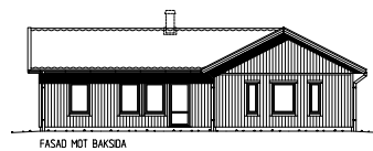
FASAD MOT BAKSIDA
