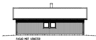
FASAD MOT VÄNSTER
