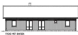
FASAD MOT BAKSIDA
